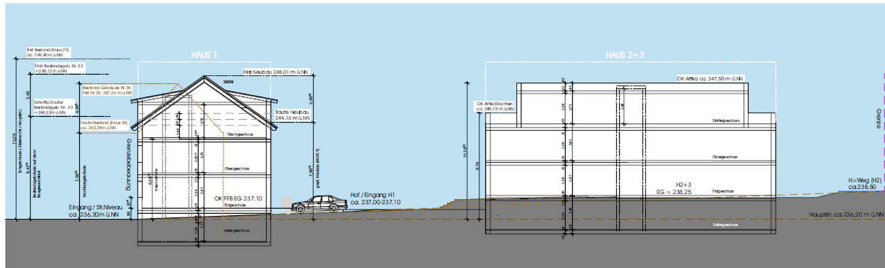
Abb. 14: Systemschnitt
